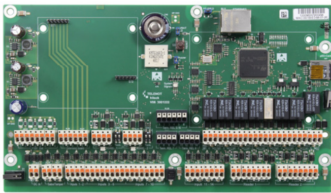
Auswerte- und Steuergerät hilock® 5500
